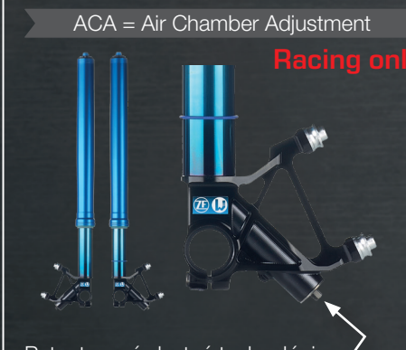
Patentovaná vlastná technológia umožňuje nastavenie vzduchovej komory pomocou šesťhranu
